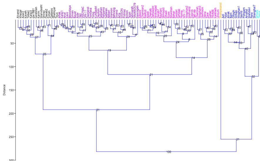
شکل ۴- گروه‌بندی ارقام های گندم نان این تحقیق براساس معیار گروه‌بندی UPGMA و با فاصله اقلیدسی Figure 4. Grouping of bread wheat varieties based upon UPGMA clustering criteria and with Euclidean distance
