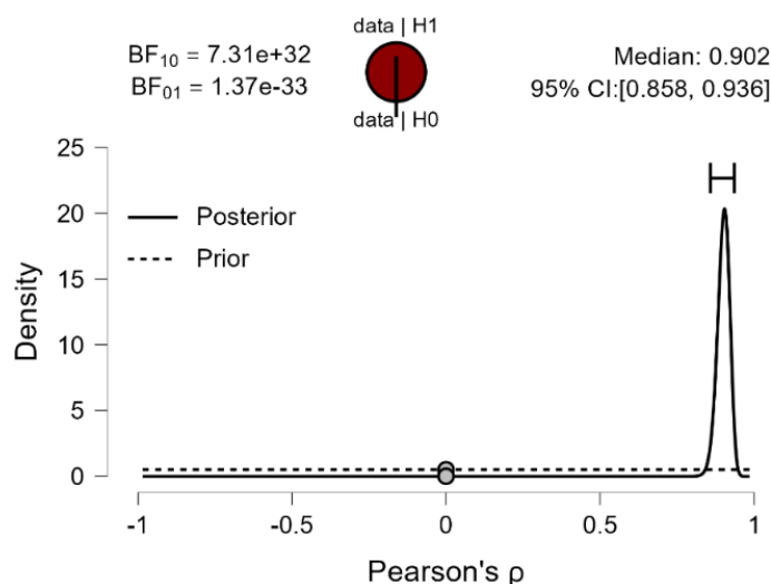
شکل ۲- نمودار خروجی برای تجزیه همبستگی بیزی دو صفت مهم وزن هزاردانه و عملکرد دانه. در این نمودار، مشخص است که توزیع پسین برای همبستگی از پیک (اوج) خیلی بیشتری نسبت به توزیع پیشین برخوردار بوده که نشان‌دهنده آگاهی ما نسبت به داده‌های مشاهده شده است.
