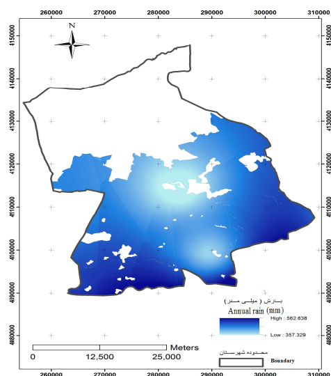
شکل ۴. نقشه برخی از متغیرهای هواشناسی در محدوده اراضی کشاورزی شهرستان آق‌قلا. Figure 4. Maps of some meteorological variables in agricultural lands of Aq-Qala township.
