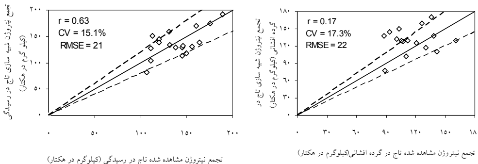
شکل ۶- مقادیر مشاهده شده و شبیه سازی شده تجمع نیتروژن در تاج در گرده افشانی و رسیدگی. خط ۱:۱ و خطوط \pm 20\% درصد نیز در شکل آورده شده اند.
