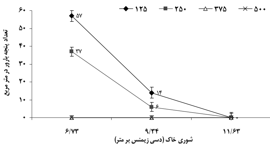
شکل ۱- اثر متقابل شوری و تراکم بوته در مترمربع بر تعداد پنجه بارور.
